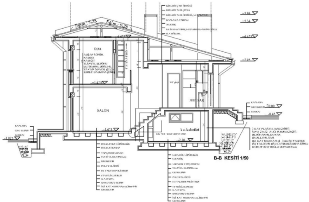
Şekil 7. İYTE Lojmanları B1 tip 90m2 kesit. Çizim: A.C. Benli, Neşe Köse, Yadigar İnşaat.
